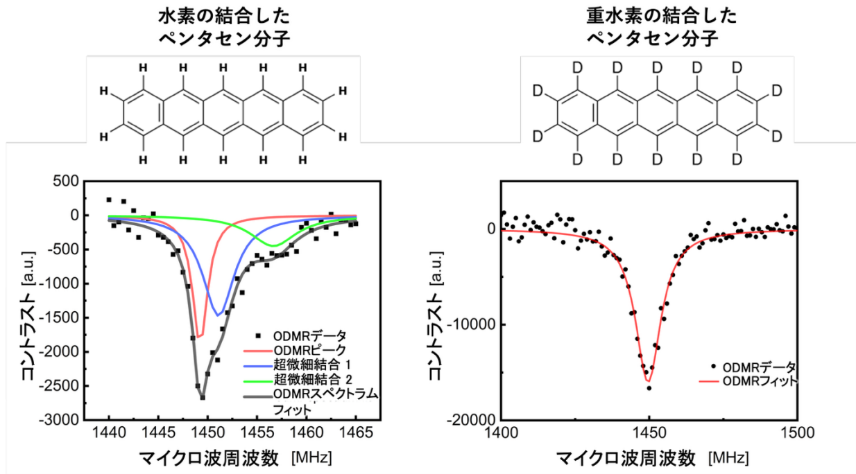
図 3. ペンタセン分子の重水素化による ODMR スペクトラムの制御
